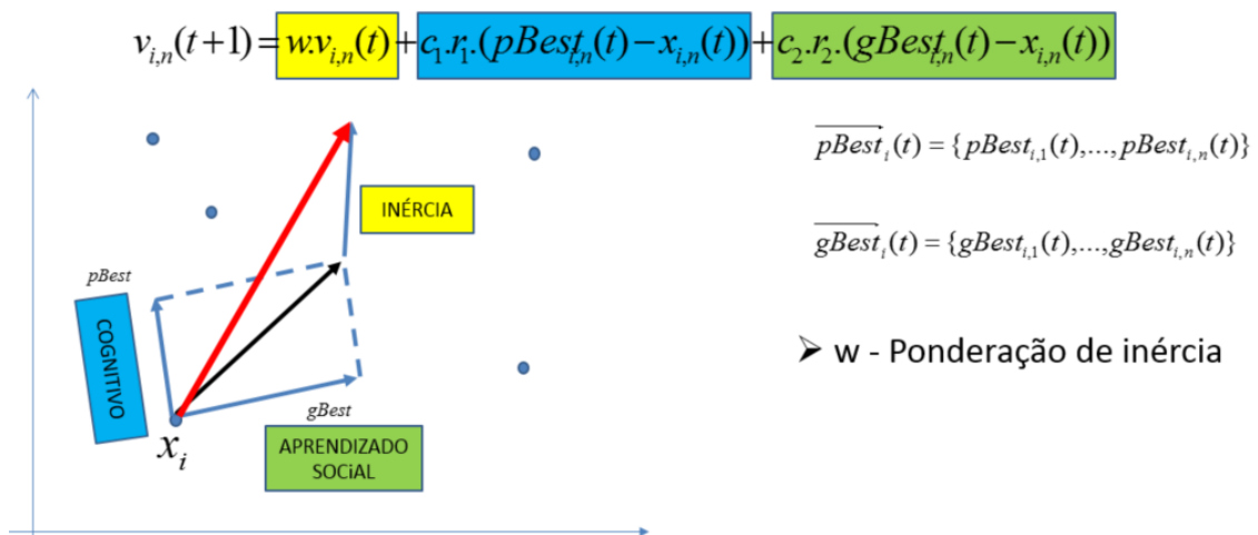
Figura 3 - Movimento da partículas do PSO
