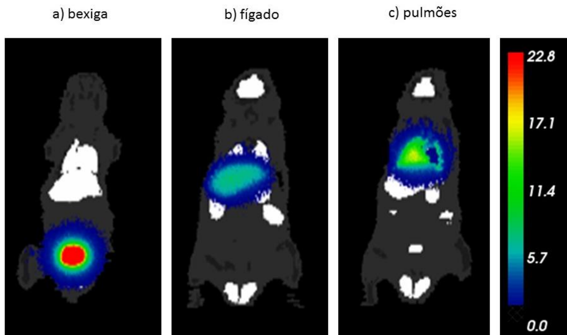
Figura 4.5 – Mapas de distribuição de energia depositada, corte coronal, em cada órgão-fonte para o radiofármaco ^{99m}\text{Tc} -Ixolaris: a) bexiga; b) fígado; c) pulmões.
